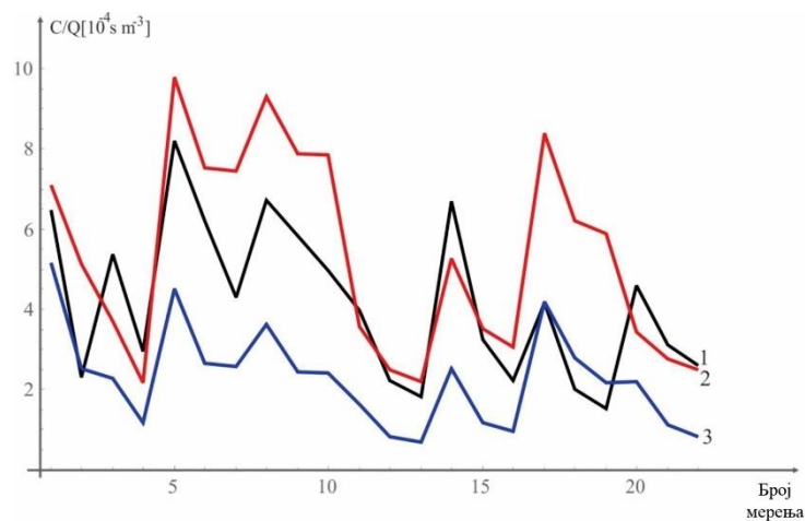
Слика 7. Поређење измерених и израчунатих вредности нормализованих концентрација: 1-мерене вредности, 2-вредности рачунате према Ојлеровом моделу, 3- вредности рачунате према Гаусовом моделу
