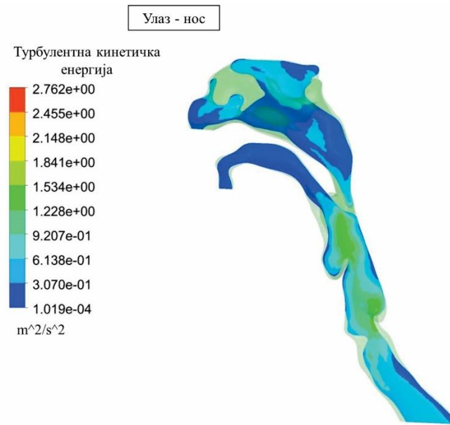
Слика 35. Случај 2 – расподела турбулентне кинетичке енергије
