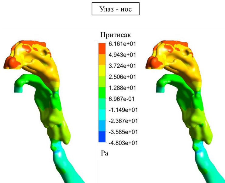
Слика 33. Случај 2 – расподела притисака
