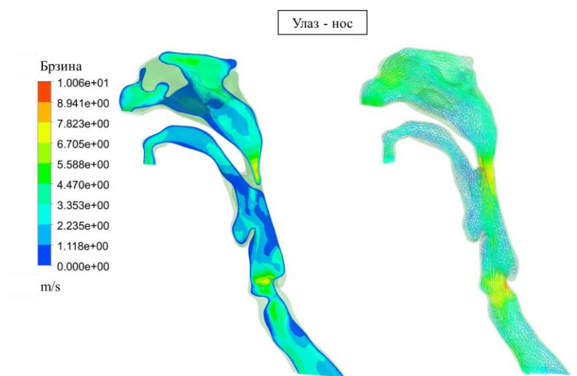
Слика 31. Случај 2 – расподела брзина
